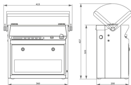
寸法図
