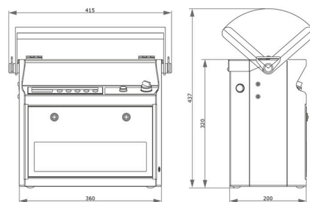
Maattekening
